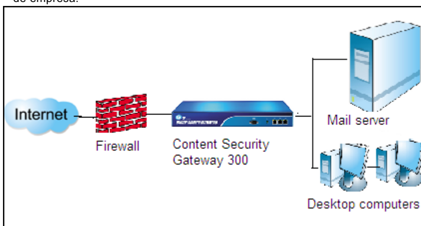
Figura 1: CP Secure Content Security Gateway 300 en la red
